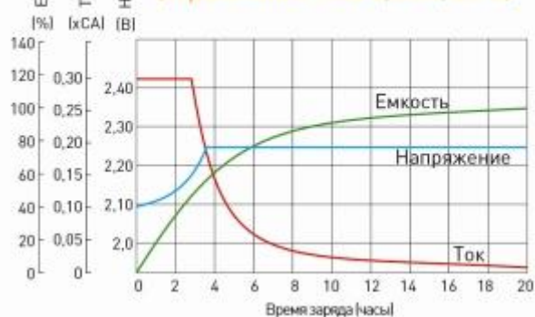
Заряд постоянным напряжением (ограничение тока 0,3С А, 25°С)
