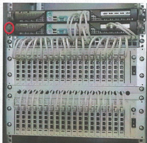
Рисунок 2 - Место пломбирования элемента системы коммутации КАТС «М-200»
